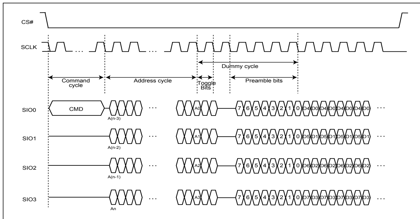
Figure 55. DTR4IO (DC=6)
